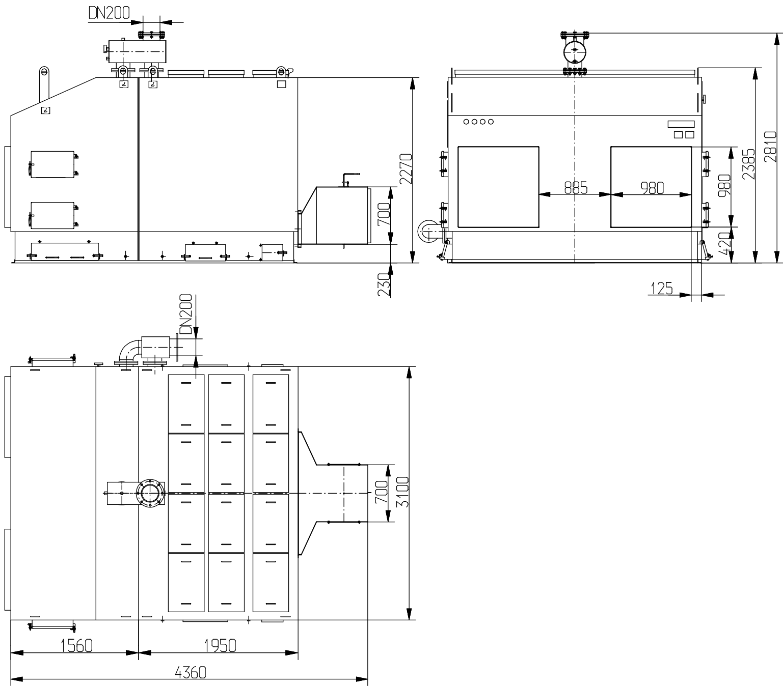
Kocioł wodny KWH-2000- wymiary.
