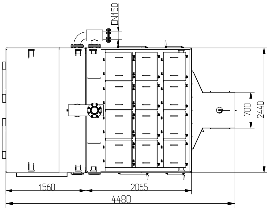
Kocioł wodny KWH-1500- wymiary.
